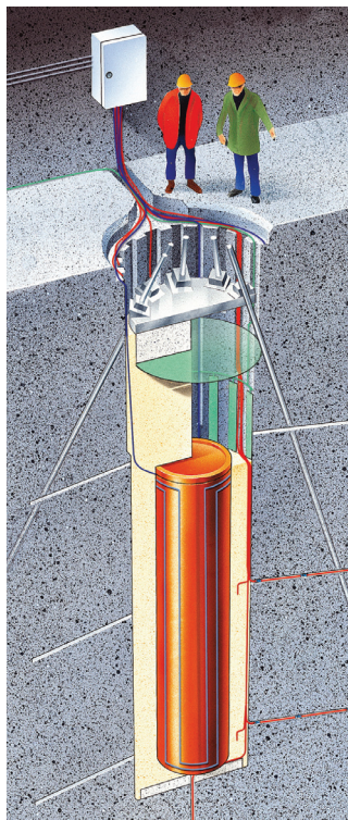
Figure 2 : Essai de récupération de conteneurs au Laboratoire sur la roche dure d'Åspö en Suède
